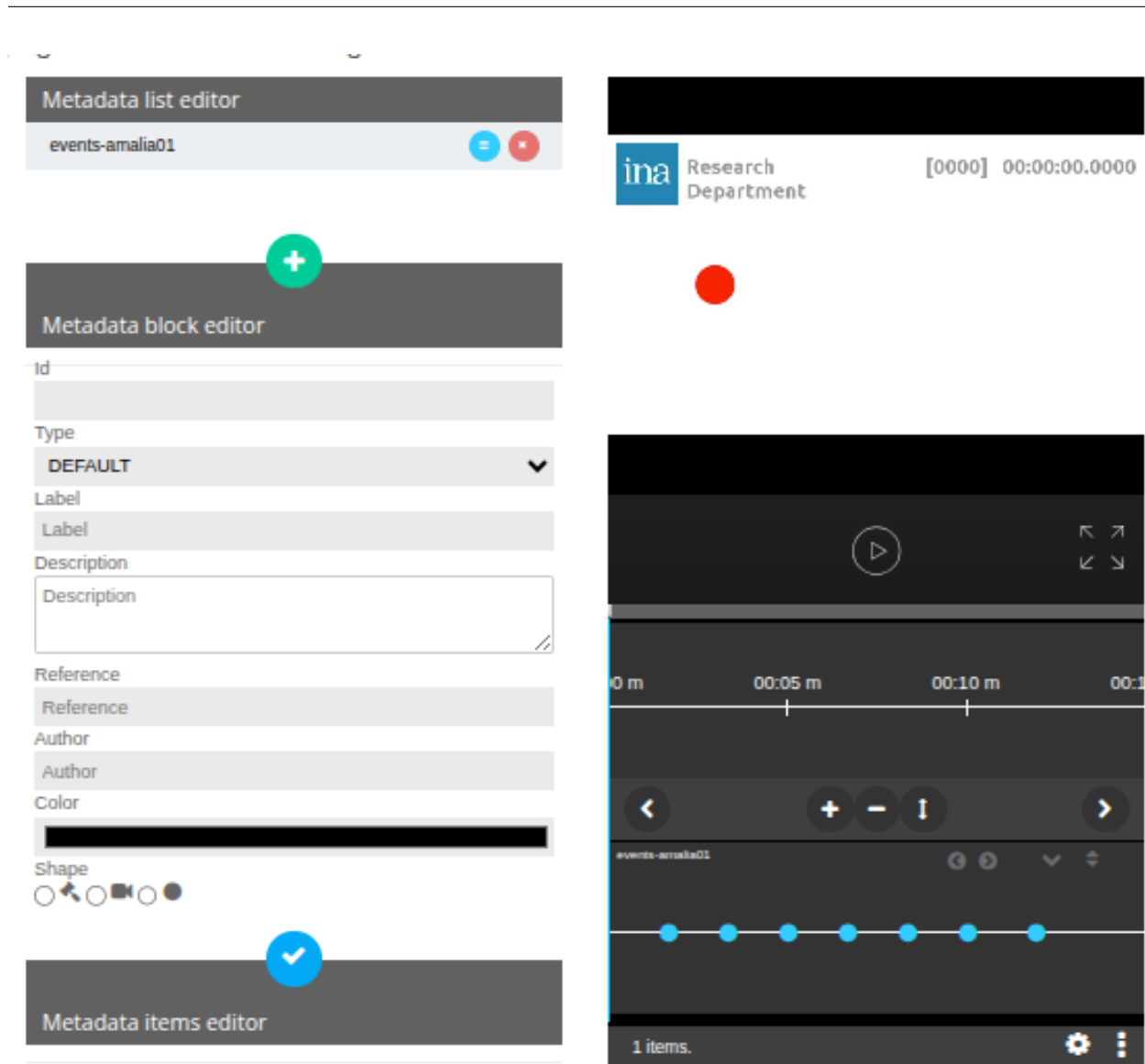
FIG. 4 : Plugin Editor dans Amalia.js 103
