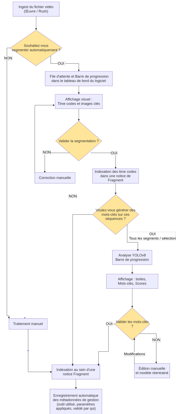
FIG. 5 : Processus de validation de l'utilisateur métier
